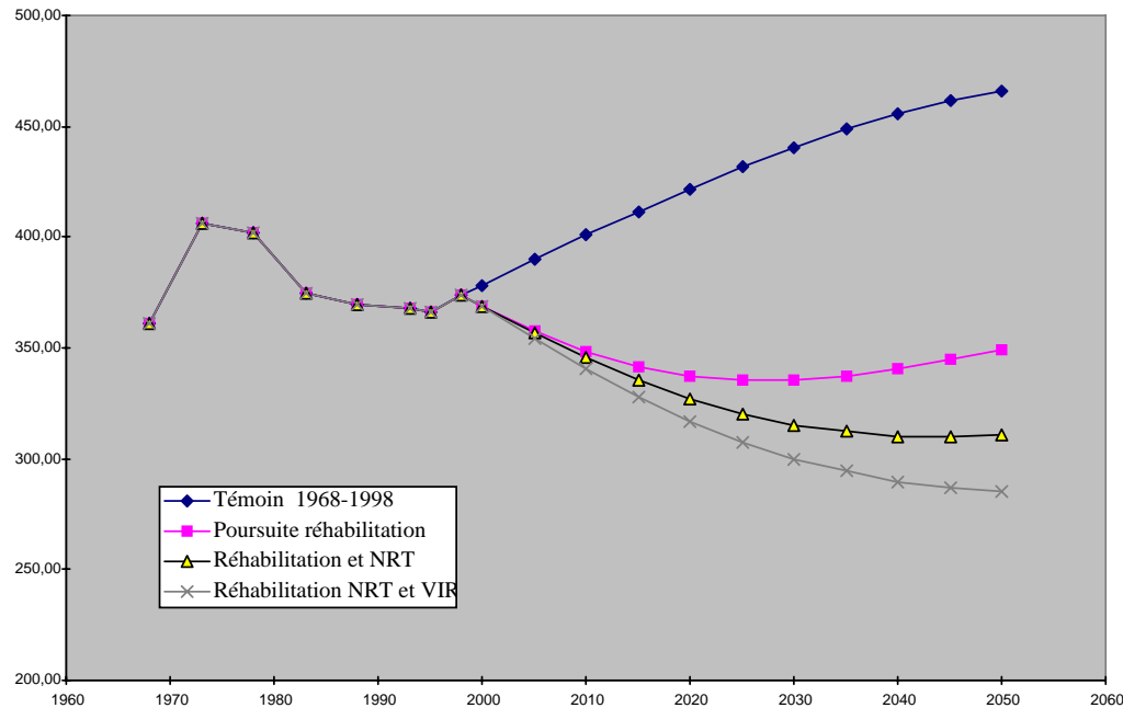
Scénarios de consommation d'énergie de chauffage du parc de résidences principales (TWh/an)
