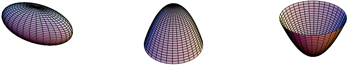
Figure 4. Surfaces à courbure positive : ellipsoïde, maximum local, minimum local.
