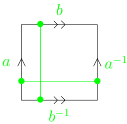
Le tore \mathbb{T}
