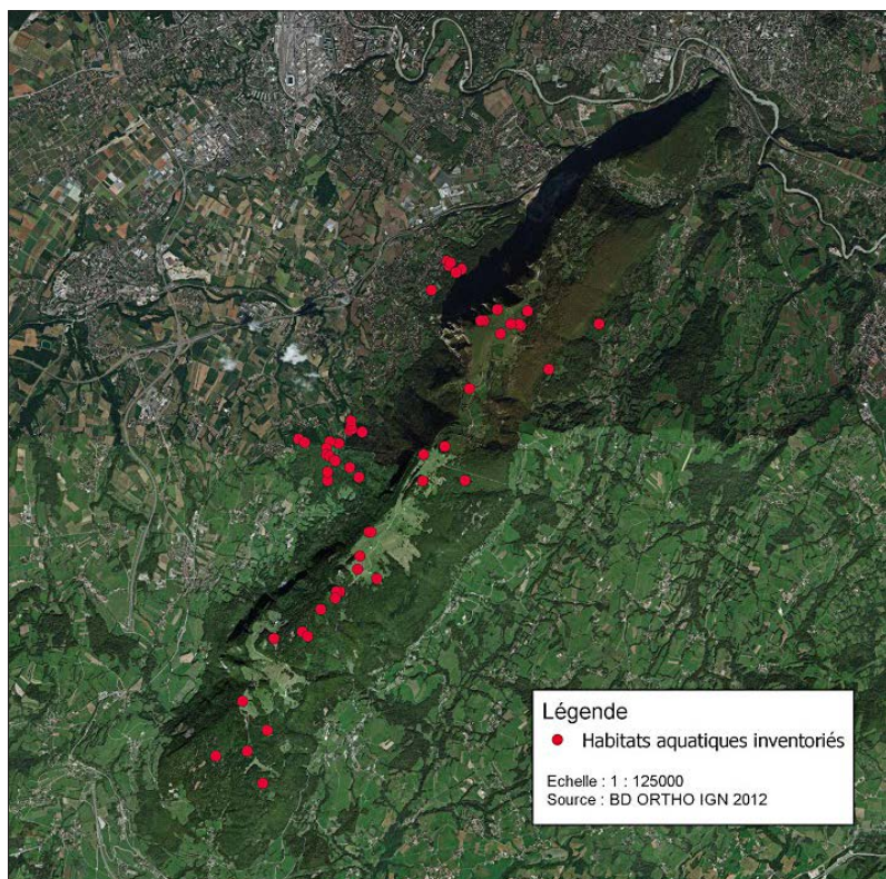
Fig. 1. Localisation de l'ensemble des sites aquatiques investigués durant ces 3 années (2011 à 2013).
