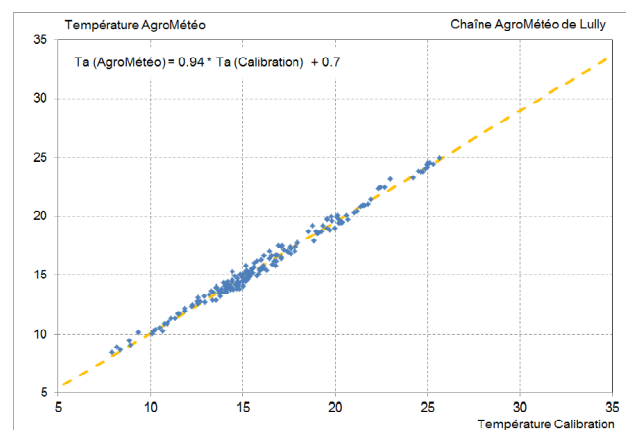
Calibration de la température T_a
