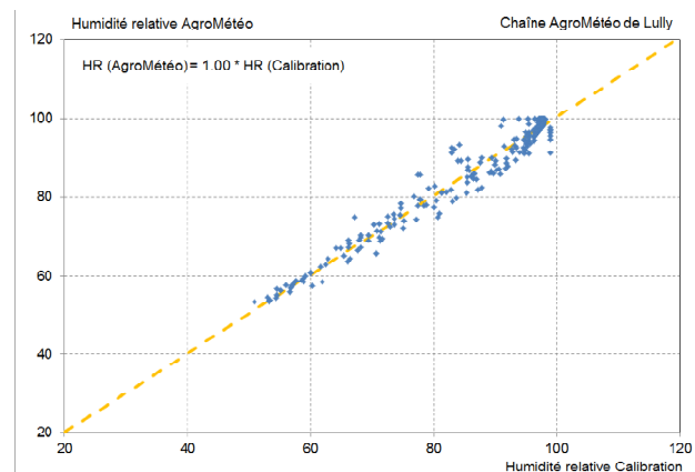
Calibration de l'humidité relative HR
